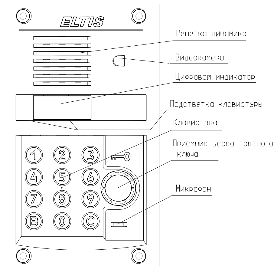
Рис.1 Внешний вид со стороны лицевой панели блока вызова DP303-RDC24.
