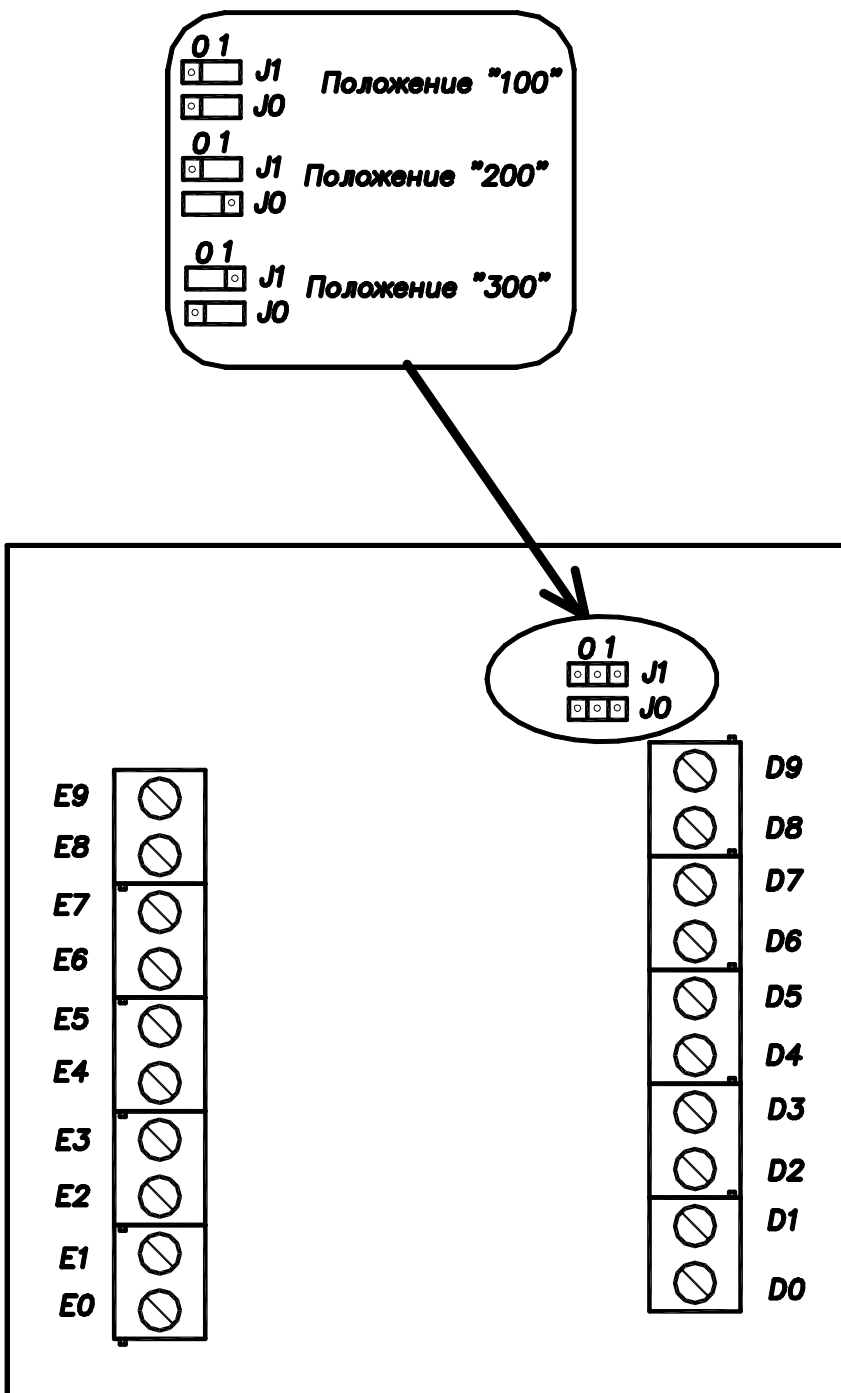
Рис.4 Установка джамперов в коммутаторе КМ100-7.
